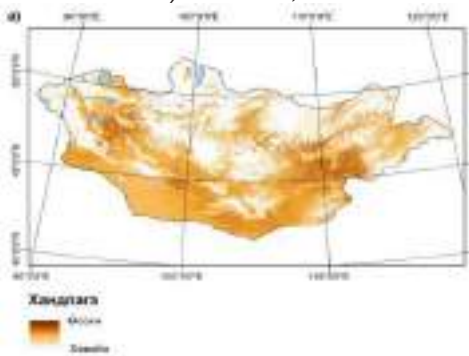
Зураг 80. 2001-2015 оны хооронд илэрсэн хөрс салхиар элэгдэх үйл явц
