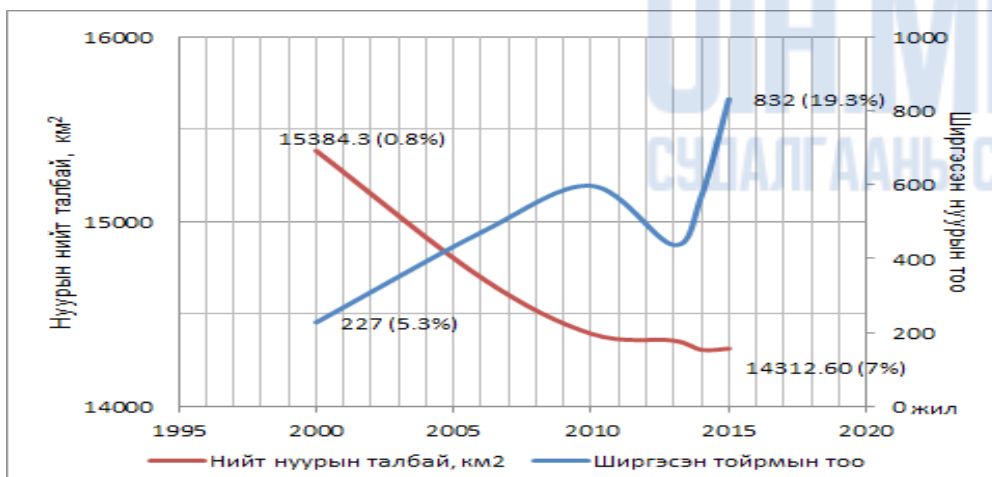
Зураг 86. Монгол орны нуурын талбай, тооны хөдлөлтүй
