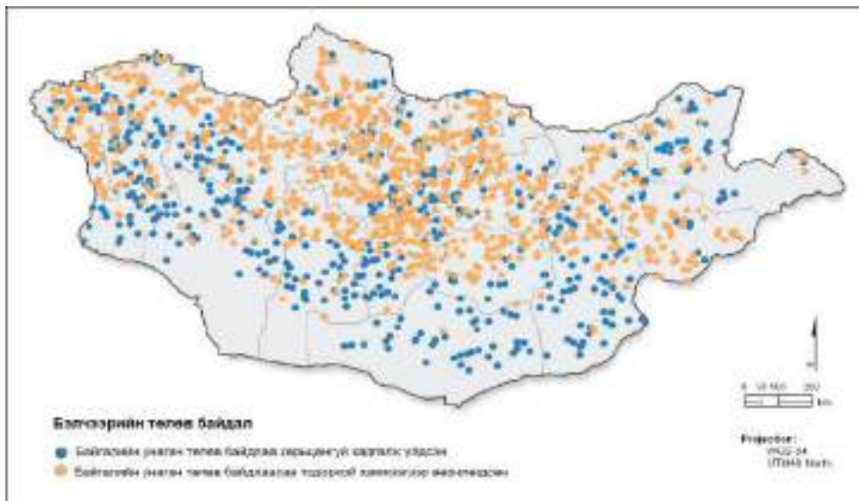
Зураг 17. Бэлчээрийн төлөв байдал (2015 он)
