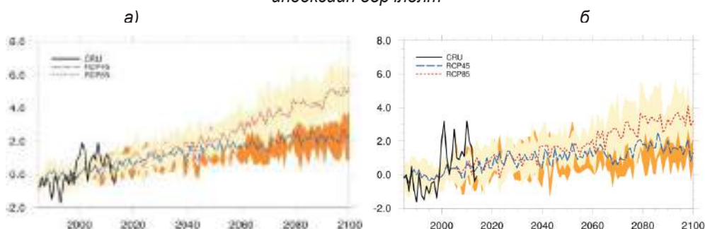
Зураг 9. Уур амьсгалын 1986-2005 оны үетэй харьцуулсан ирээдүйн ган болон зудын индексийн өөрчлөлт
